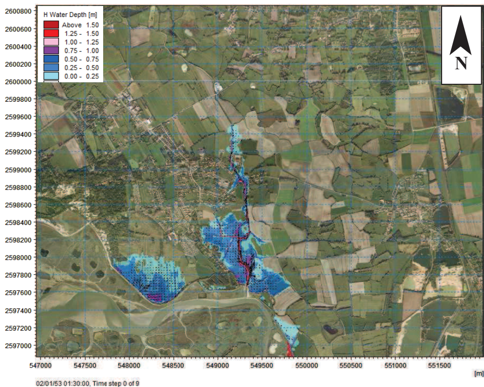
Figure 8-330: Apparition des premiers débordements (30 minutes avant la pleine-mer), aléa T100
